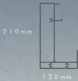
Cadre
