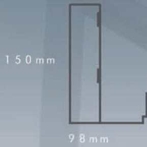
Cadre
